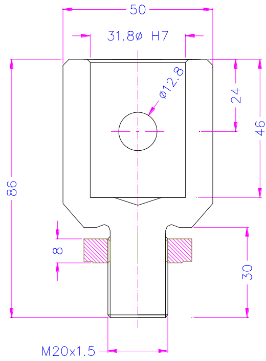
THS892-318-M20x1.5
